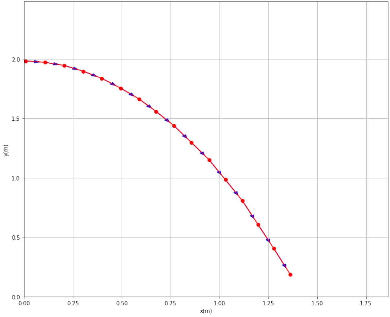
Tracé des vecteurs vitesse
